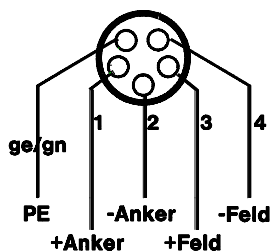
Motorkabel 808X1XE geschirmt
